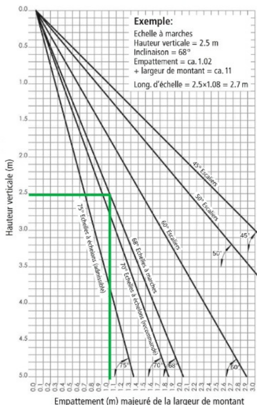
Diagramme pour le calcul de l'empatement
